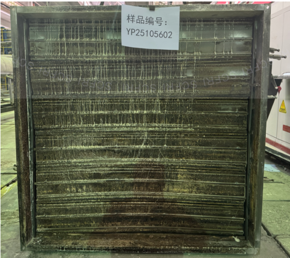
照片 2 耐火性能试验结束后试件情况
